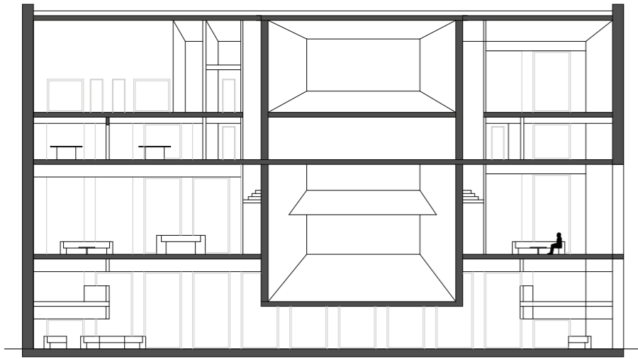
Querschnitt 1:400
