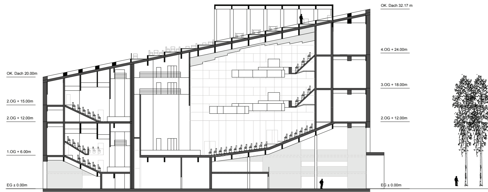
Längsschnitt 1:400
