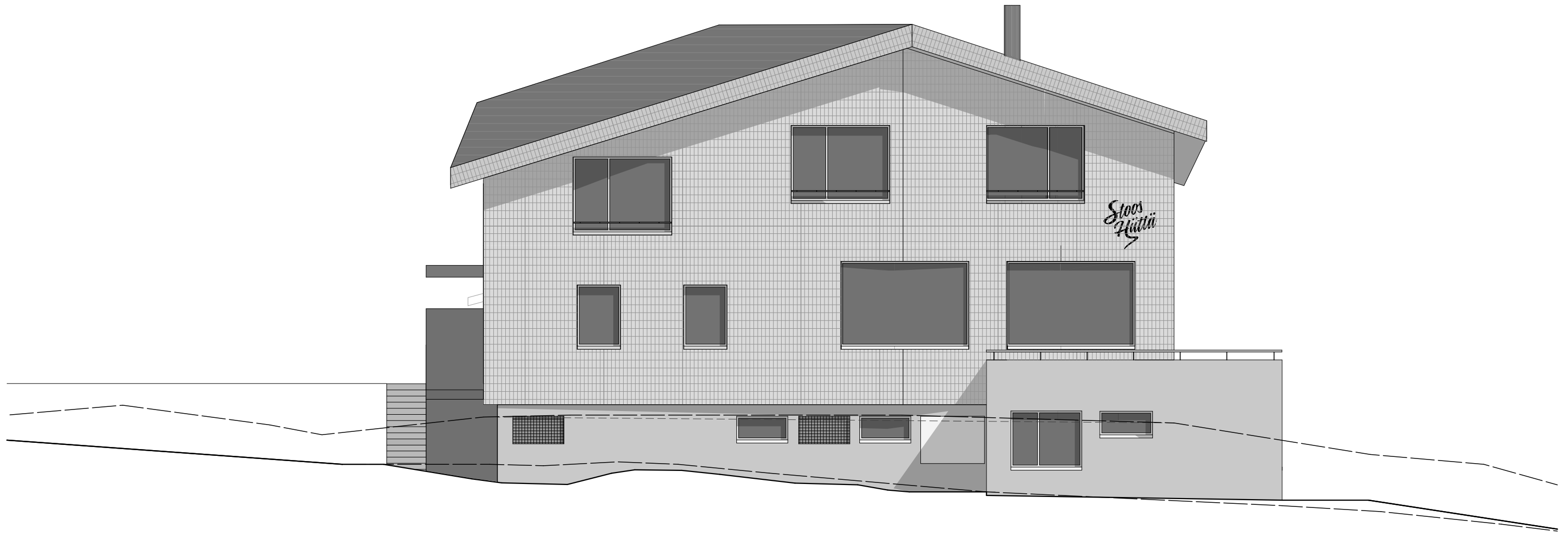
Nordfassade | 1:100
