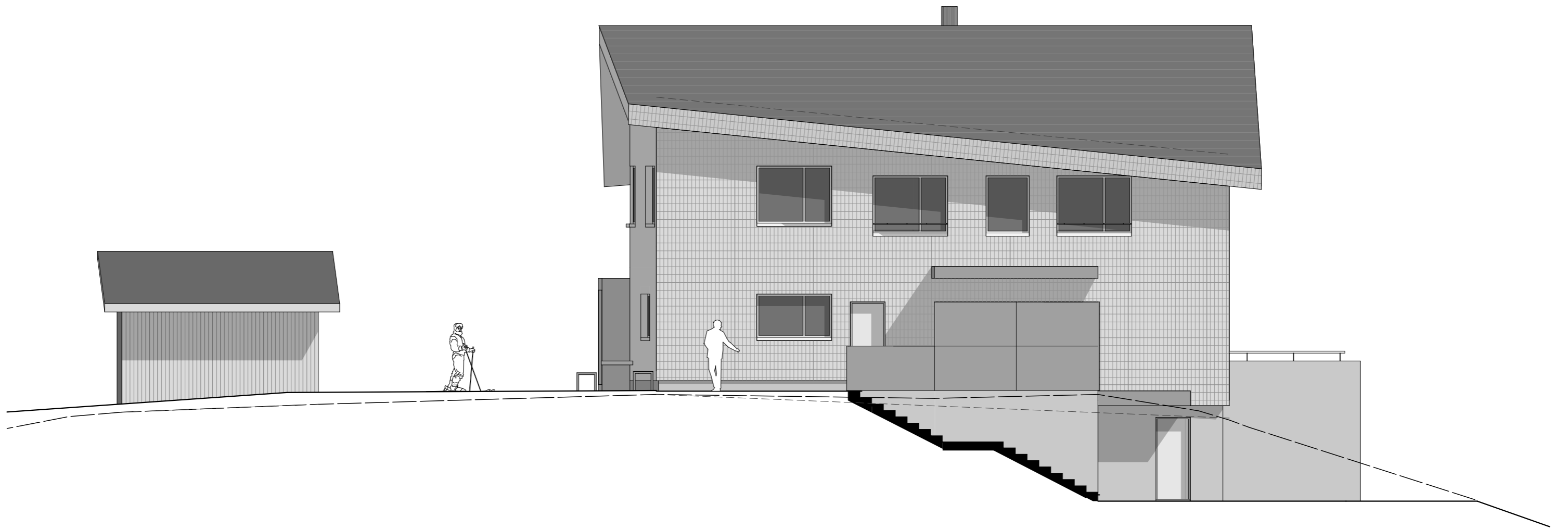
Ostfassade | 1:100
