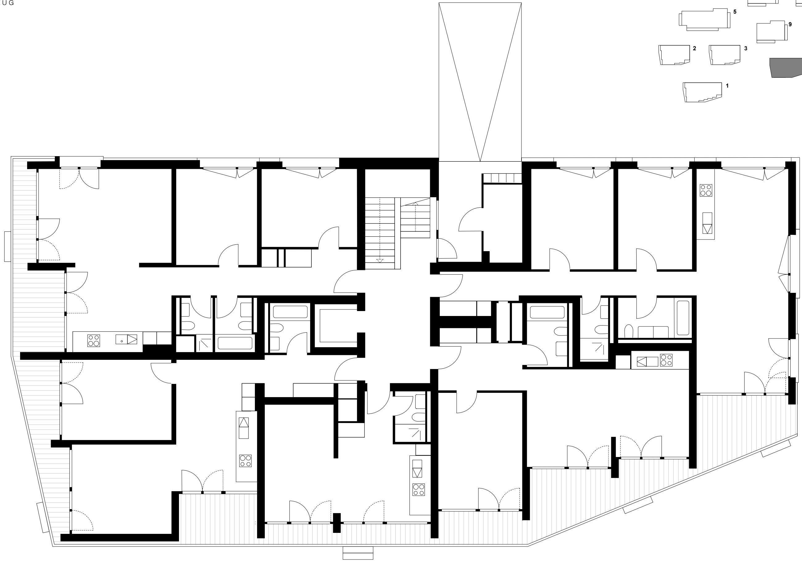
GRUNDRISS ERDGESCHOSS HAUS 4
