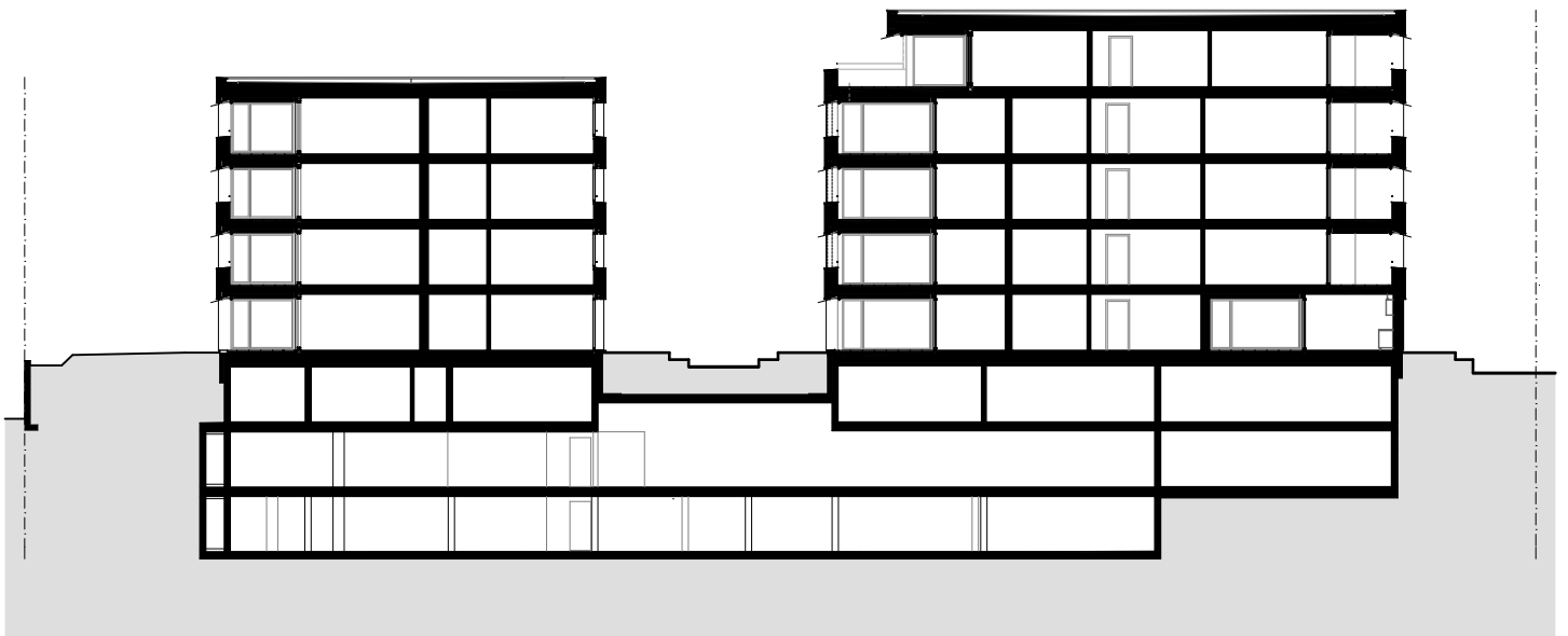
SCHNITT HAUS C / B
