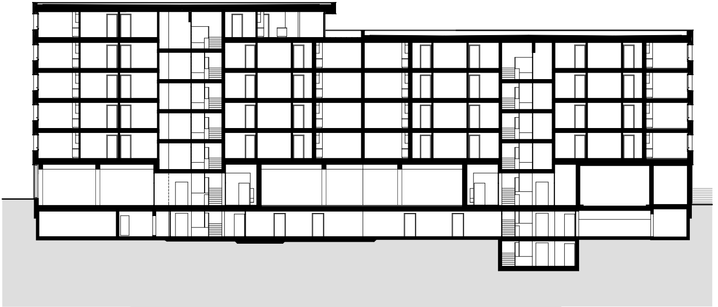
SCHNITT HAUS A
