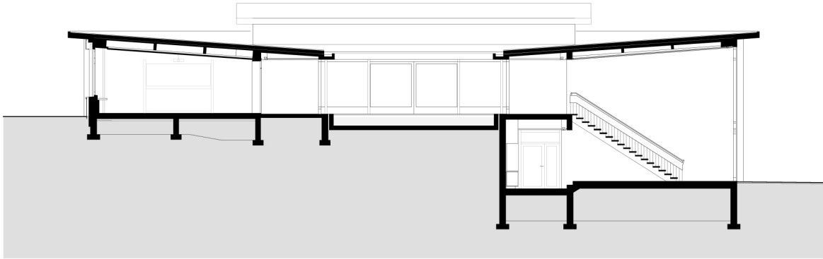
Querschnitt B-B
