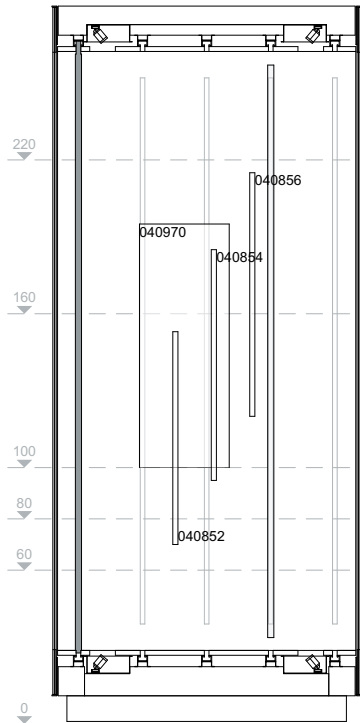
COUPE AA'
