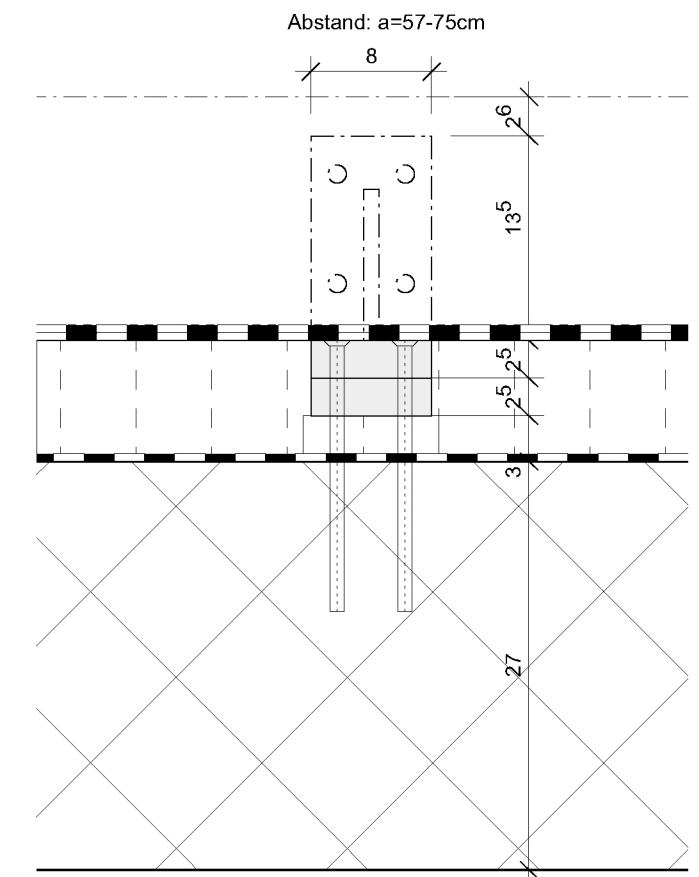
Längsschnitt
