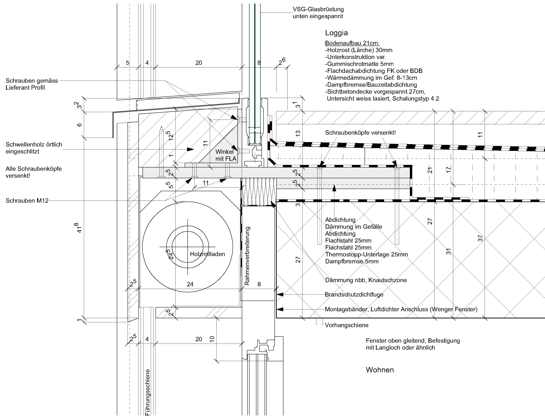
Querschnitt
