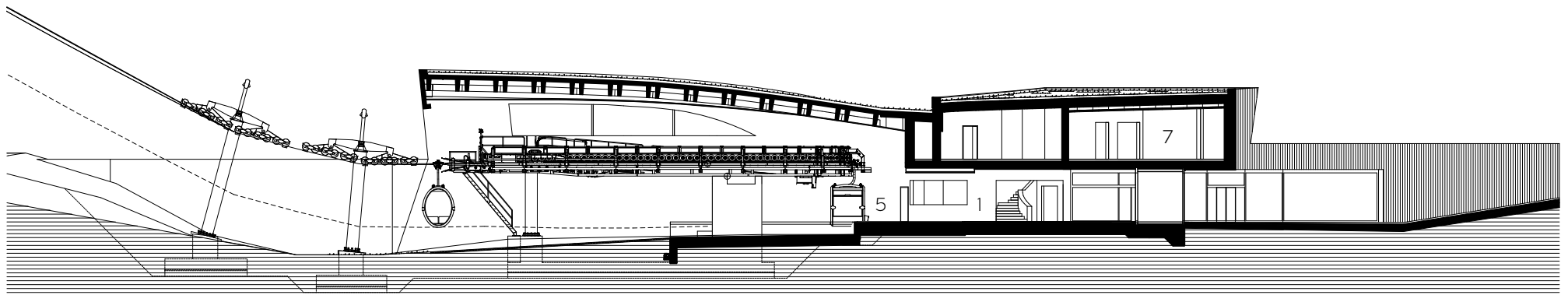
Schnitt B
