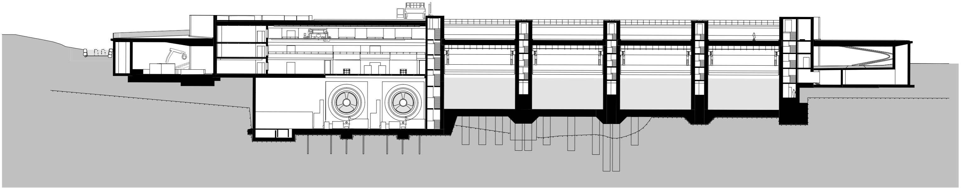
1:500 Schnitt_Wehranlage
