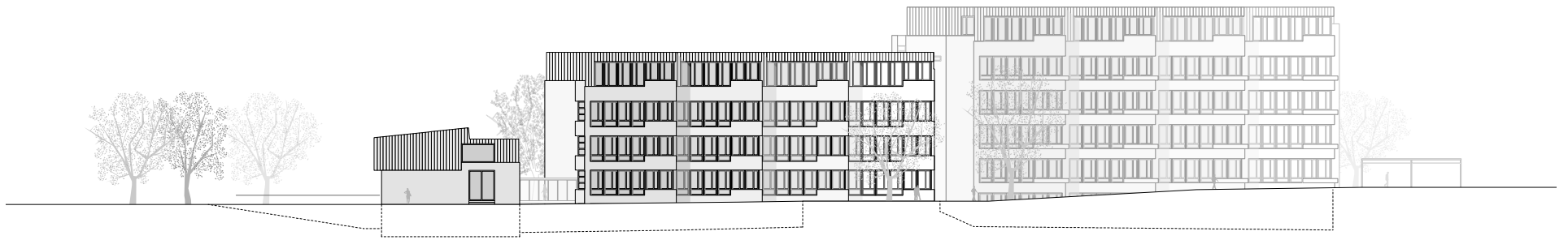
Ansicht Ost
