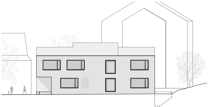
Ansicht Südost
