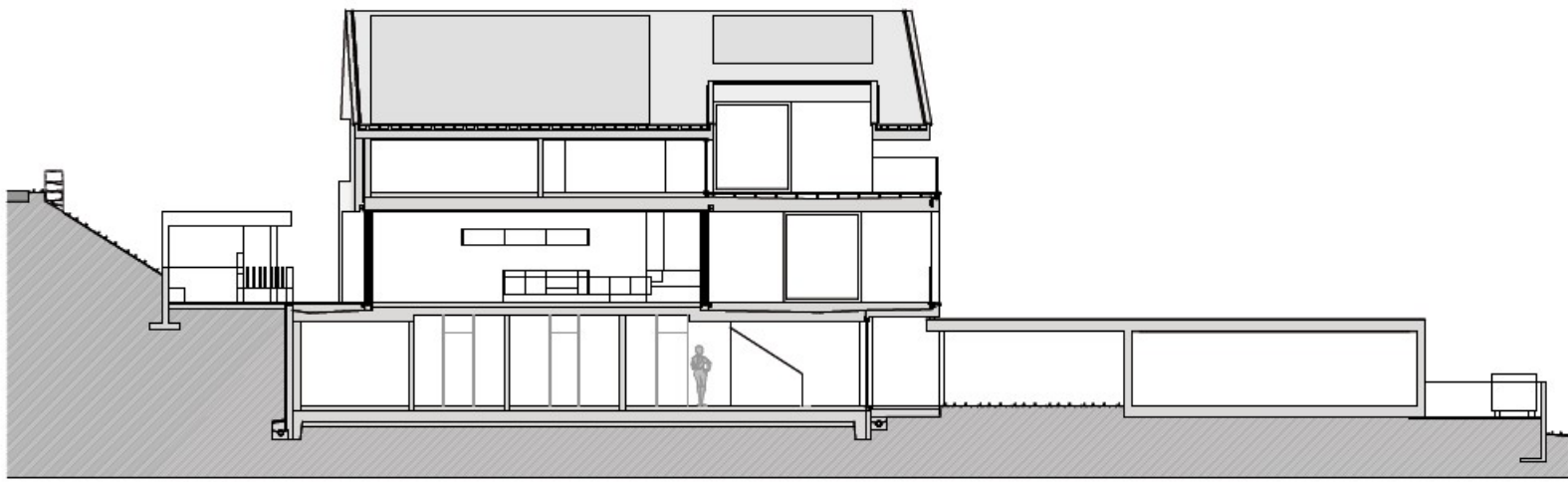
Schnitt B-B
