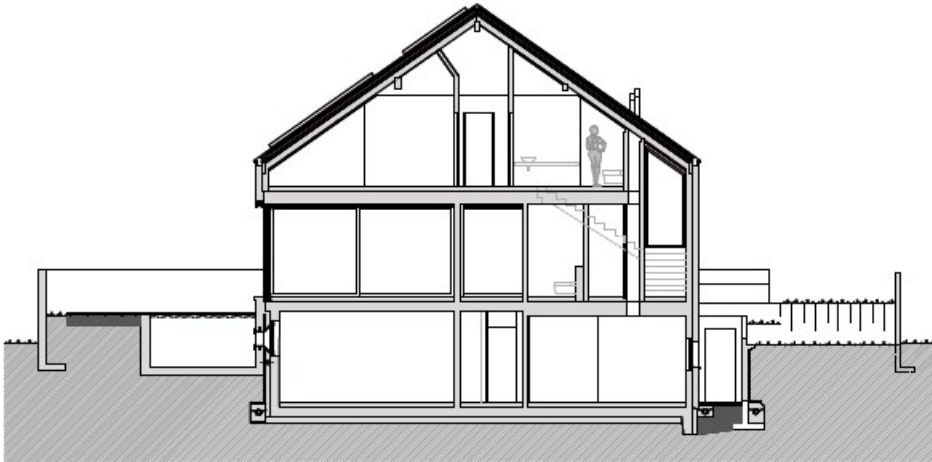
Schnitt A-A
