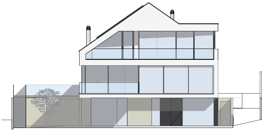
Ost Fassade
