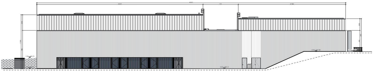
FACADE EST
