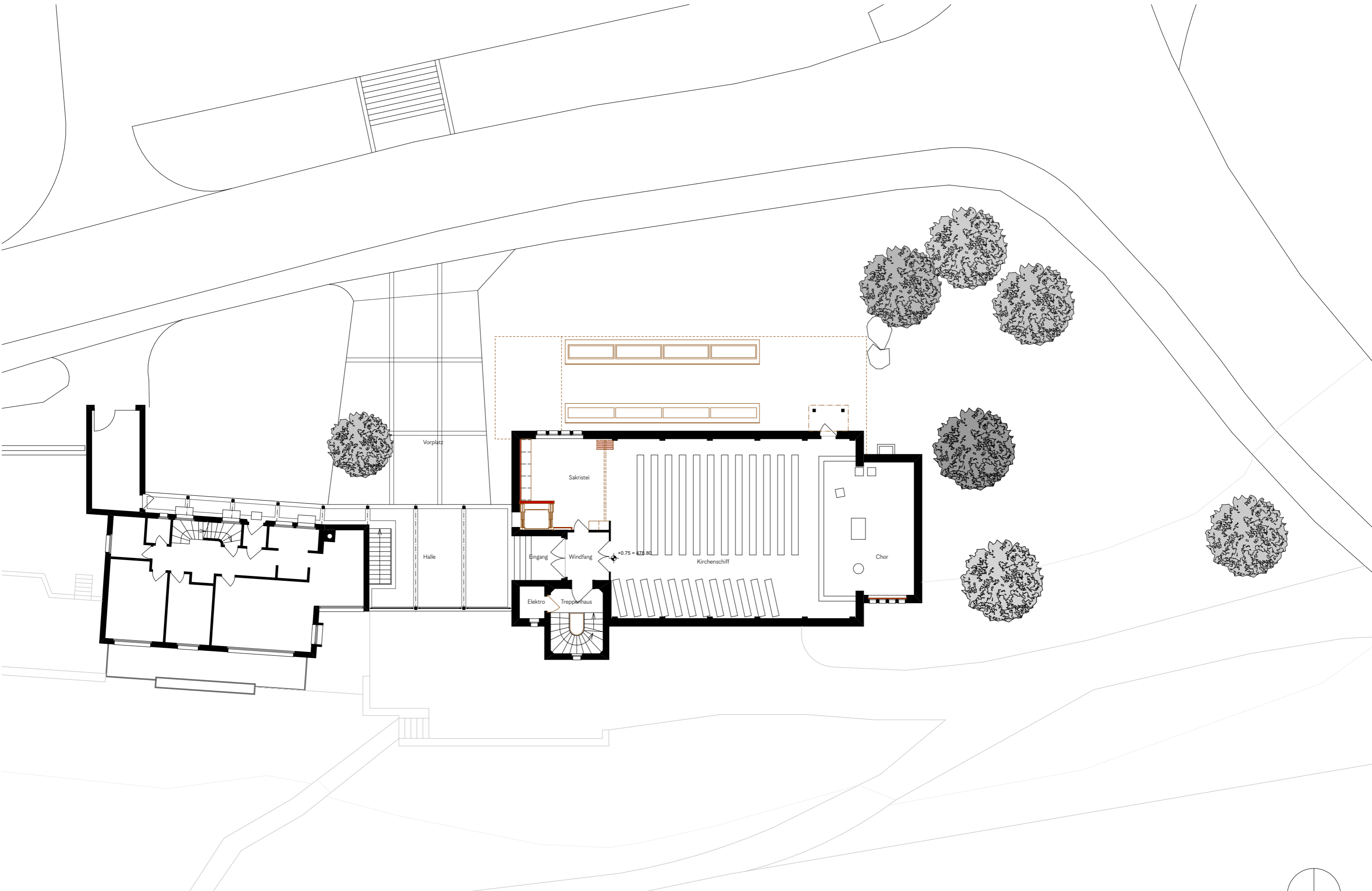
Grundriss EG 1:200
