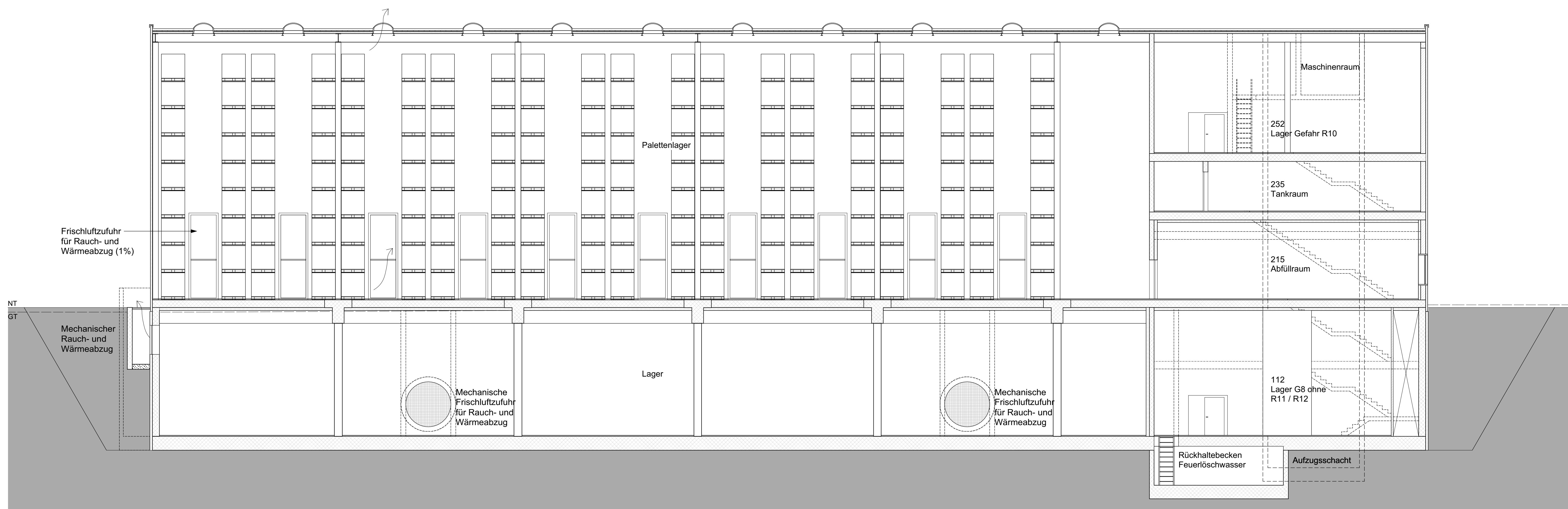
Schnitt a-a
