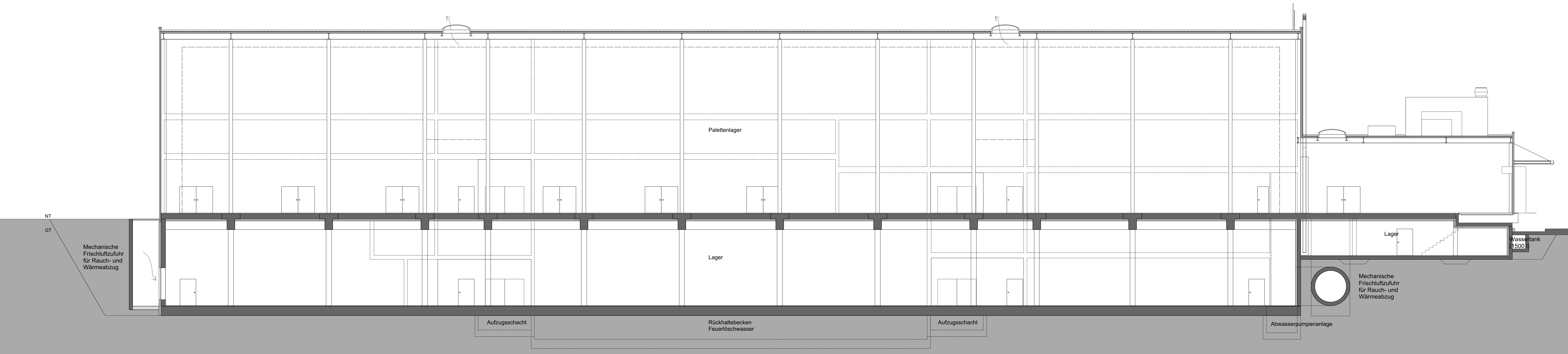
Schnitt b-b
