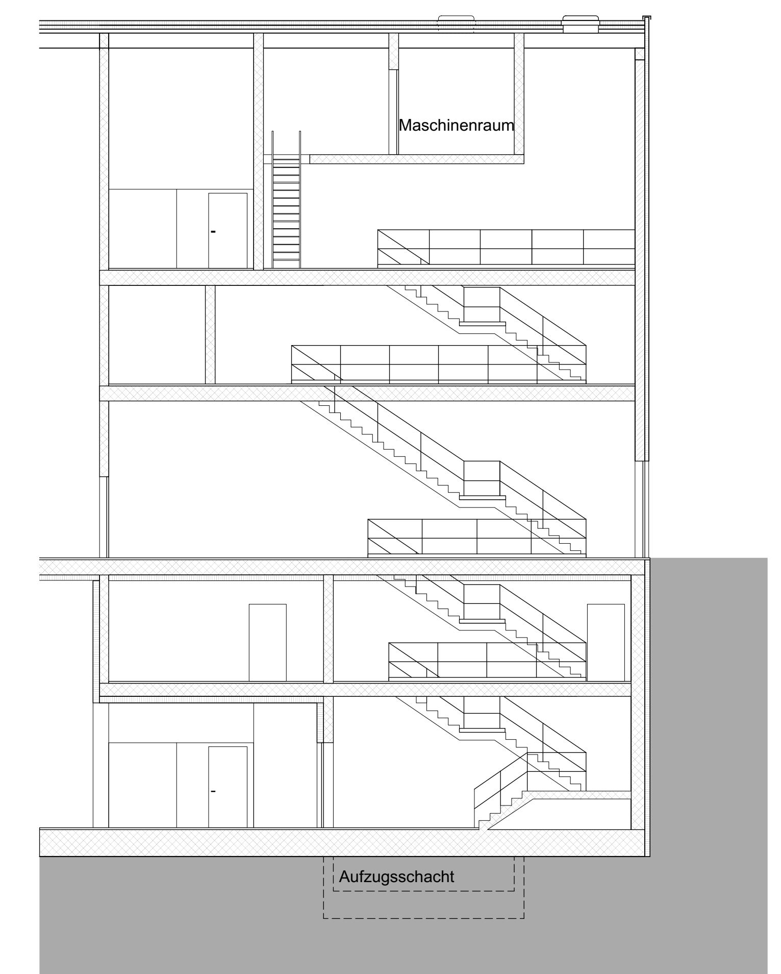
Schnitt durch Treppenhaus
