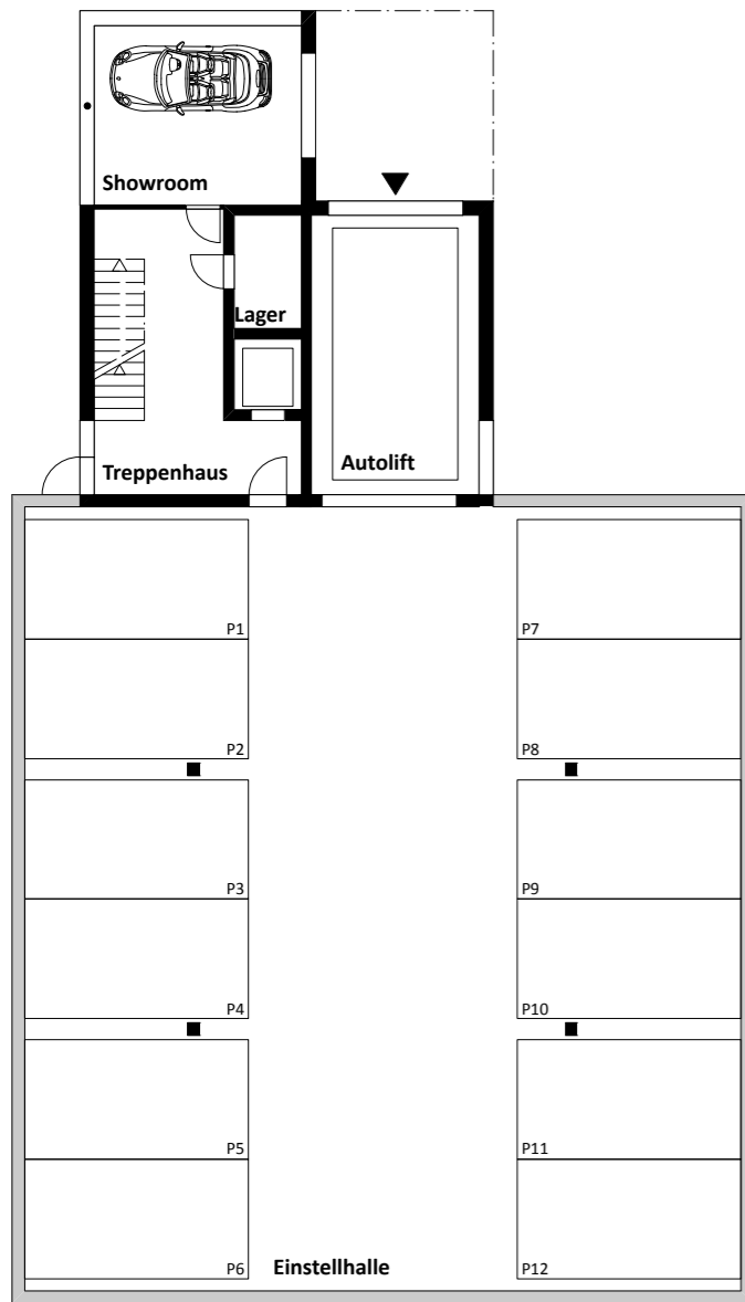
ERDGESCHOSS 1:200
