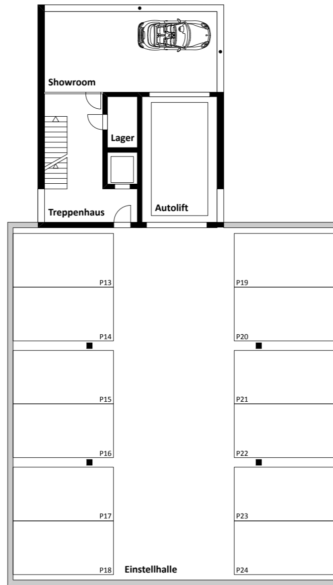
1./2. OBERGESCHOSS 1:200
