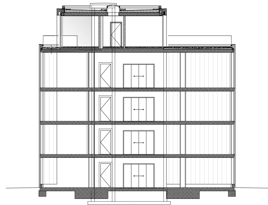
SCHNITT A-A 1:200
