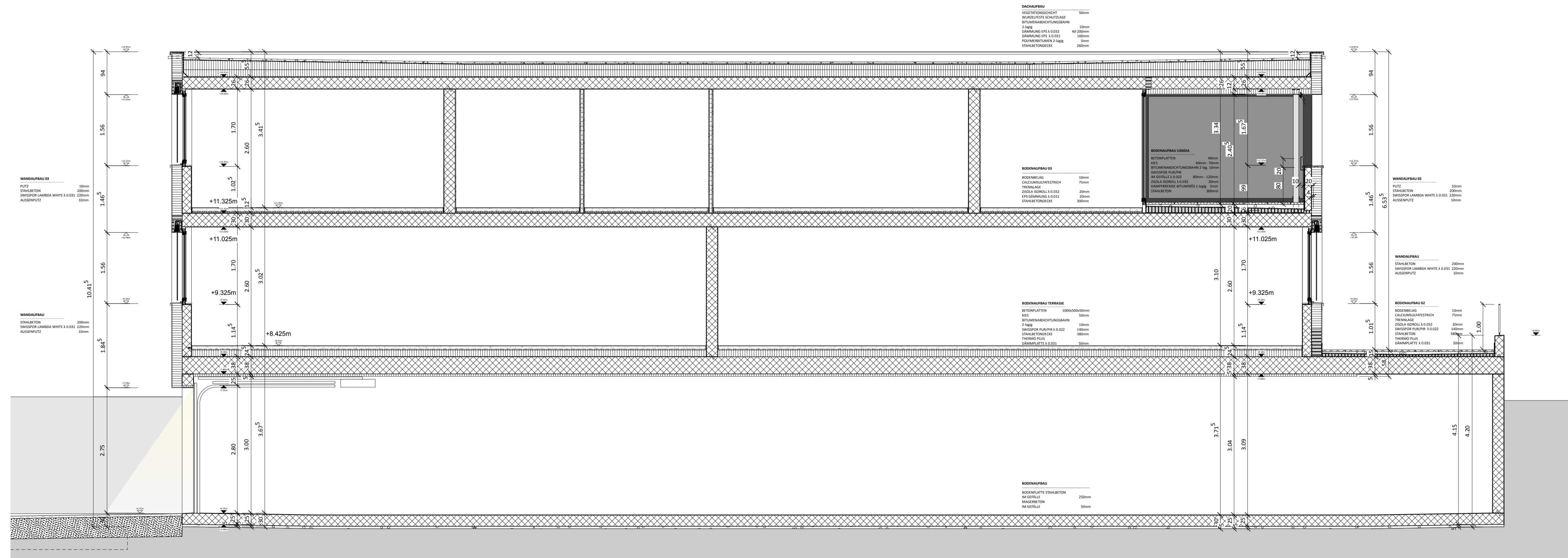
QUERSCHNITT 1:50
