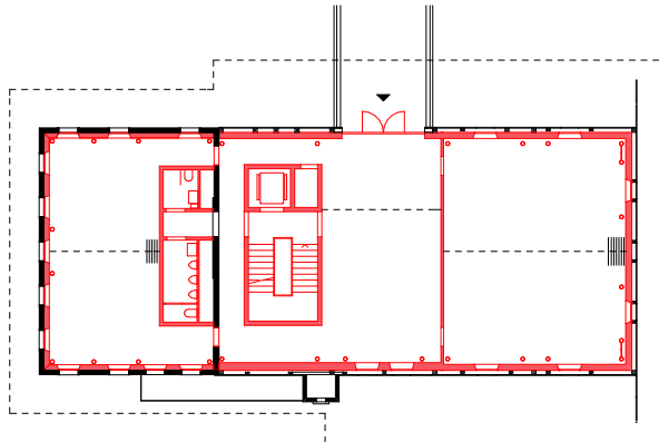
1ER ÉTAGE
