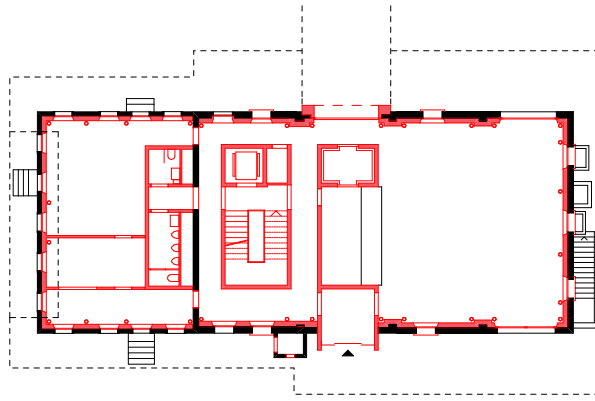
REZ-DE-CHAUSSÉE
