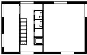
1ER ÉTAGE
