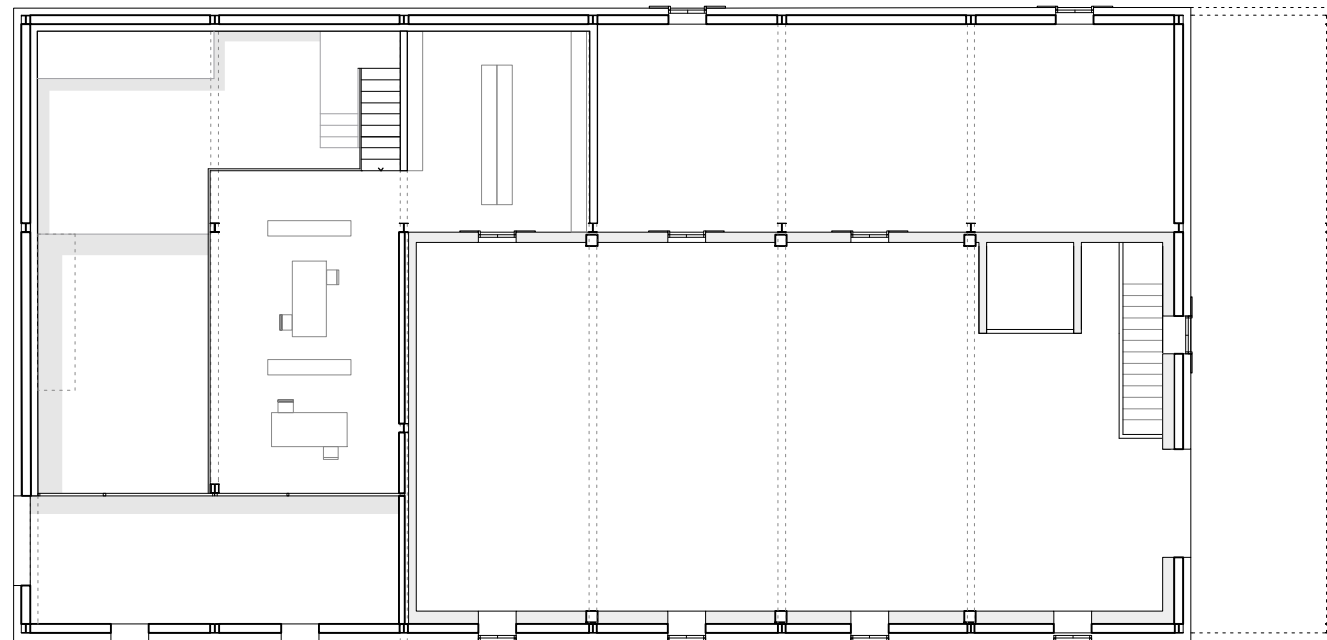
Obergeschoss 1:200
