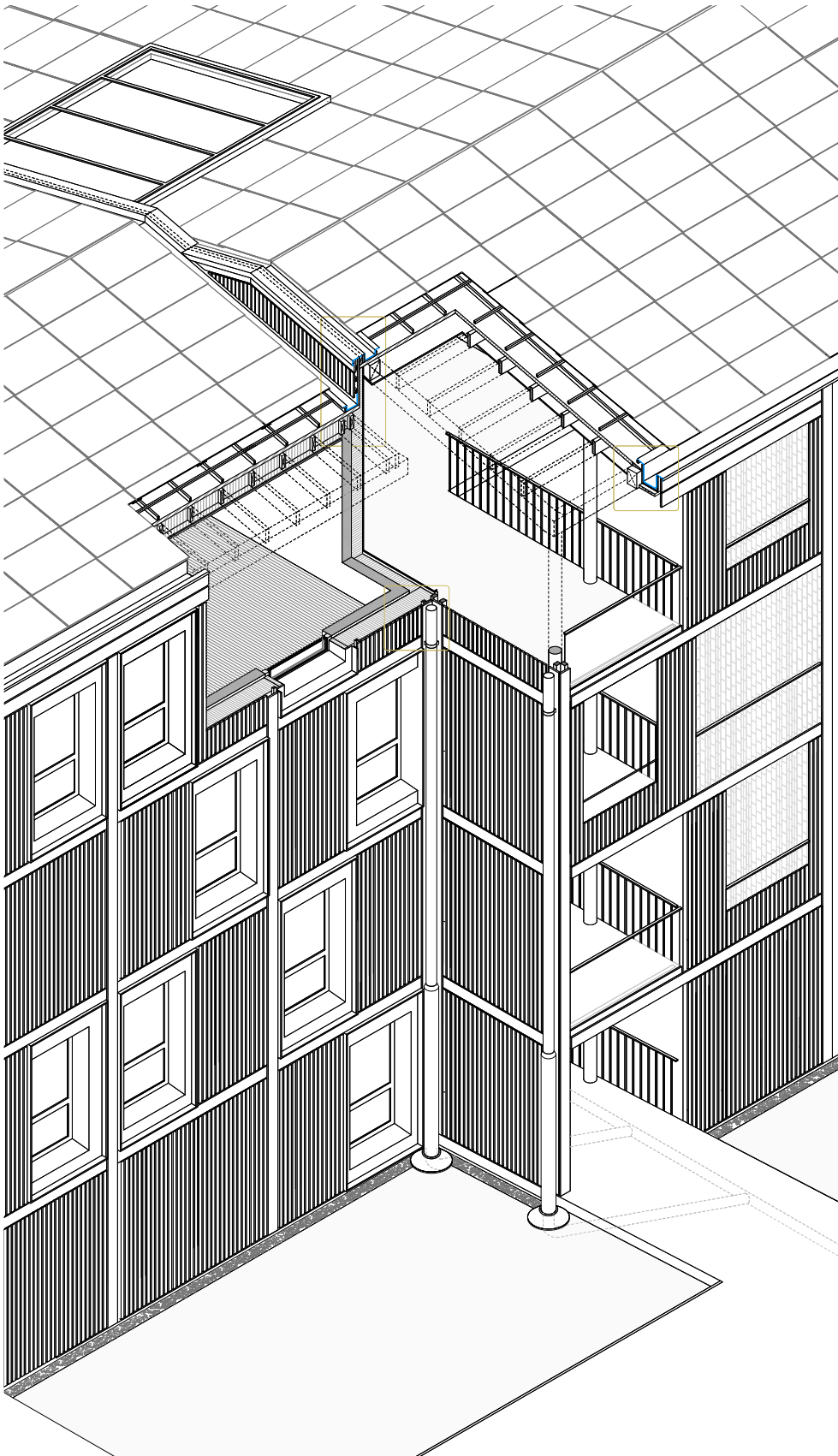
Axonométrie de la structure
