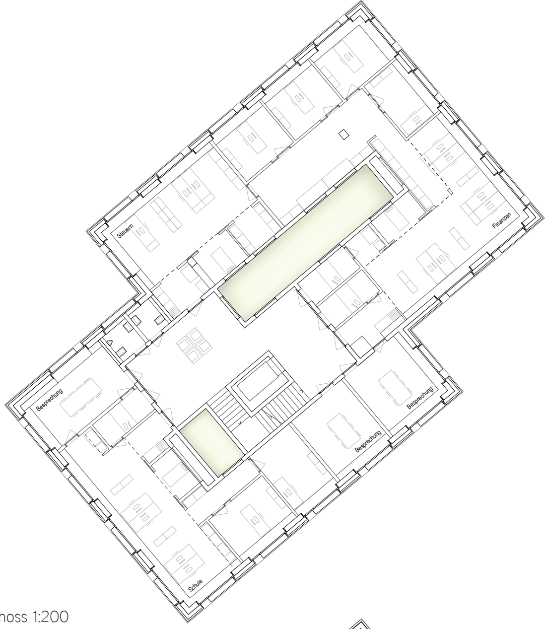
1. Obergeschoss 1:200
