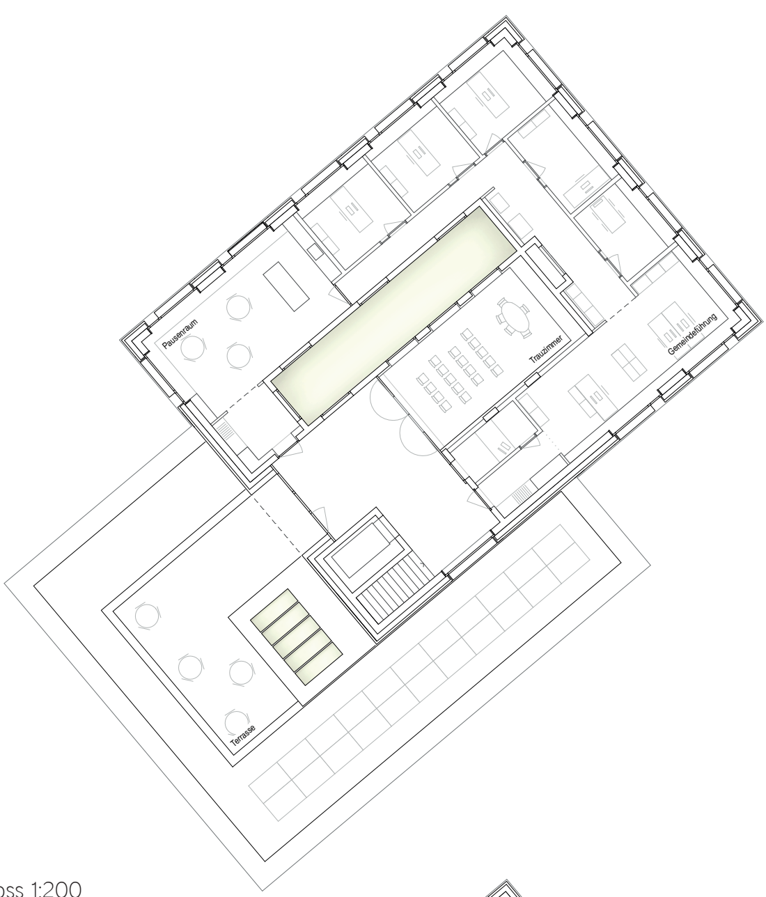
Dachgeschoss 1:200
