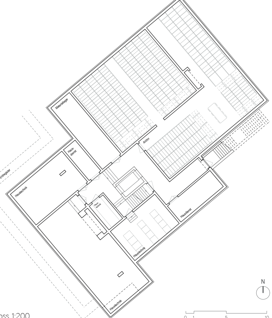
Untergeschoss 1:200
