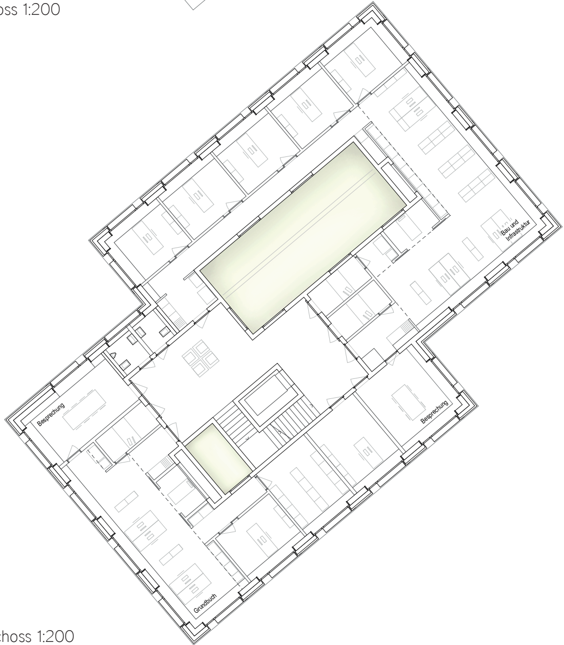
3. Obergeschoss 1:200
