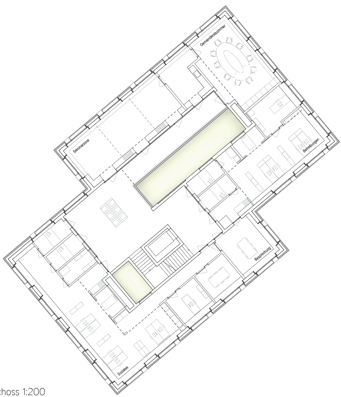
2. Obergeschoss 1:200
