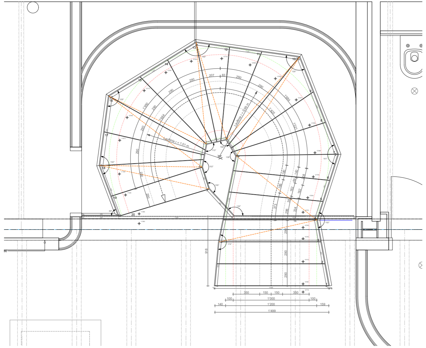
Grundriss Konstruktion 1:30
