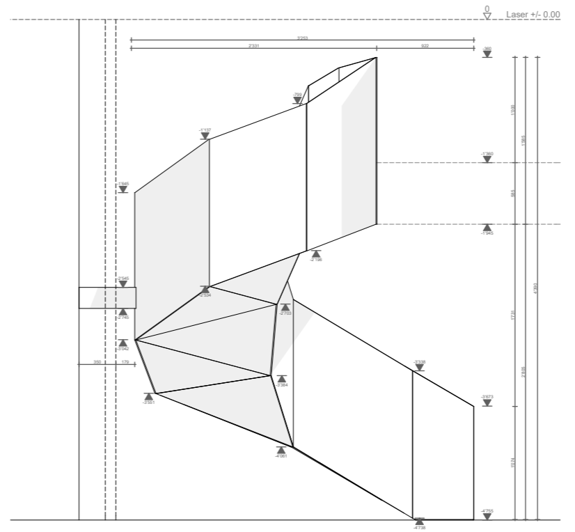
Ansichten Treppe 1:50
