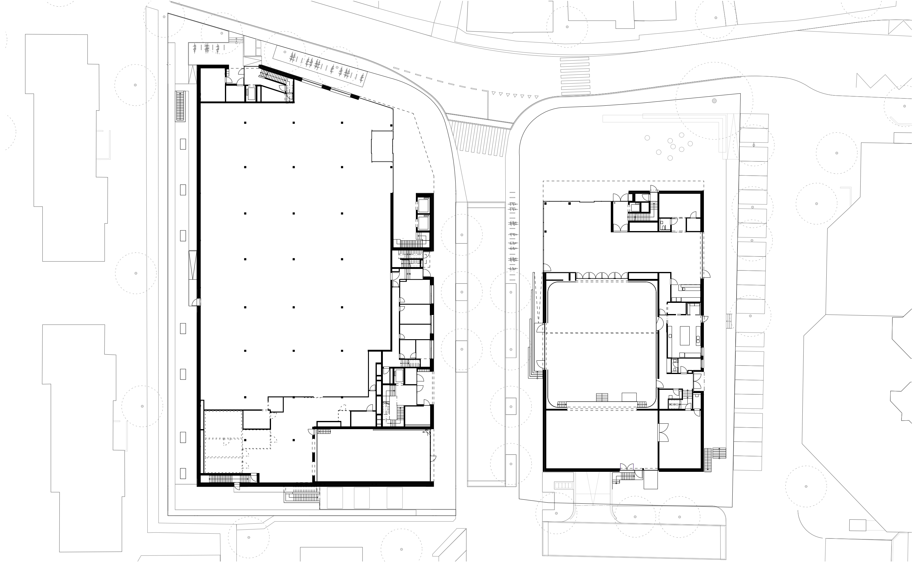
GRUNDRISS ERDGESCHOSS
