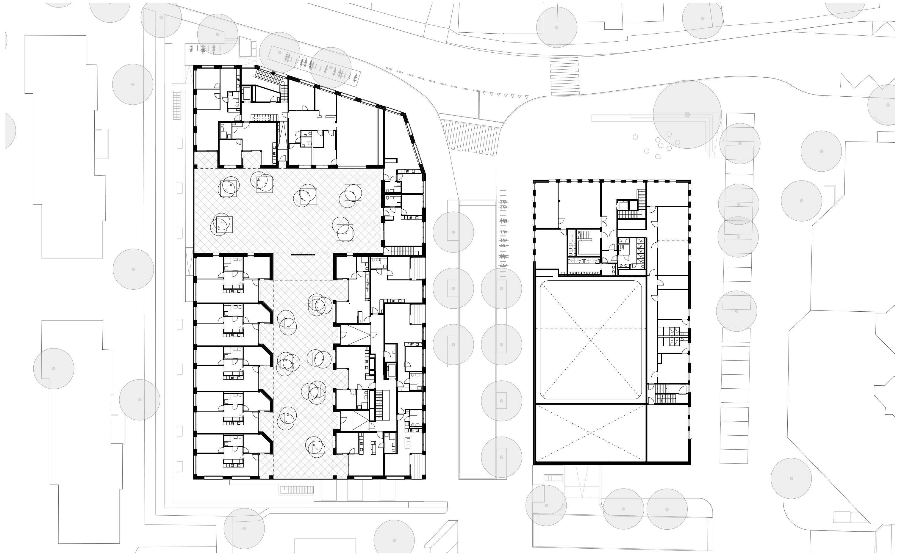
GRUNDRISS 1.OBERGESCHOSS
