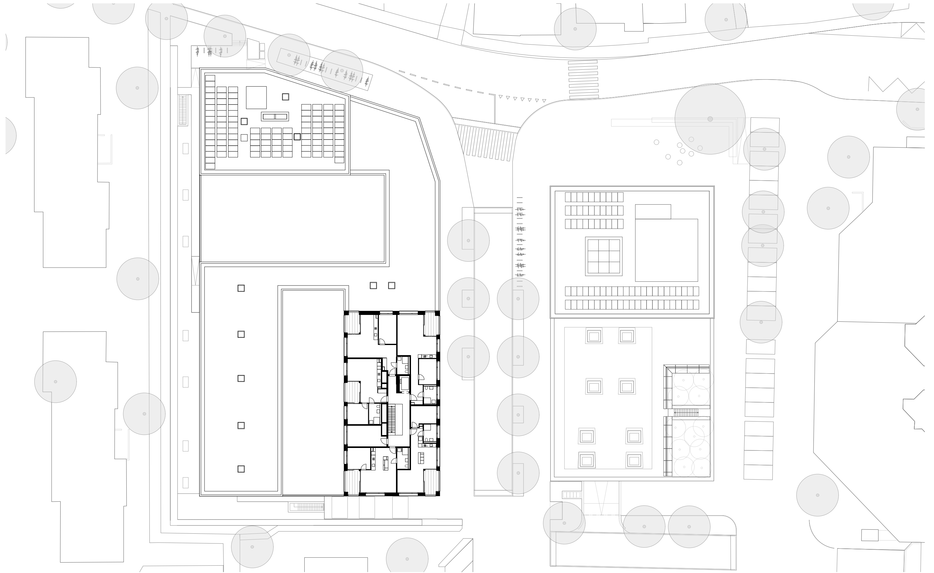
GRUNDRISS 4.OBERGESCHOSS
