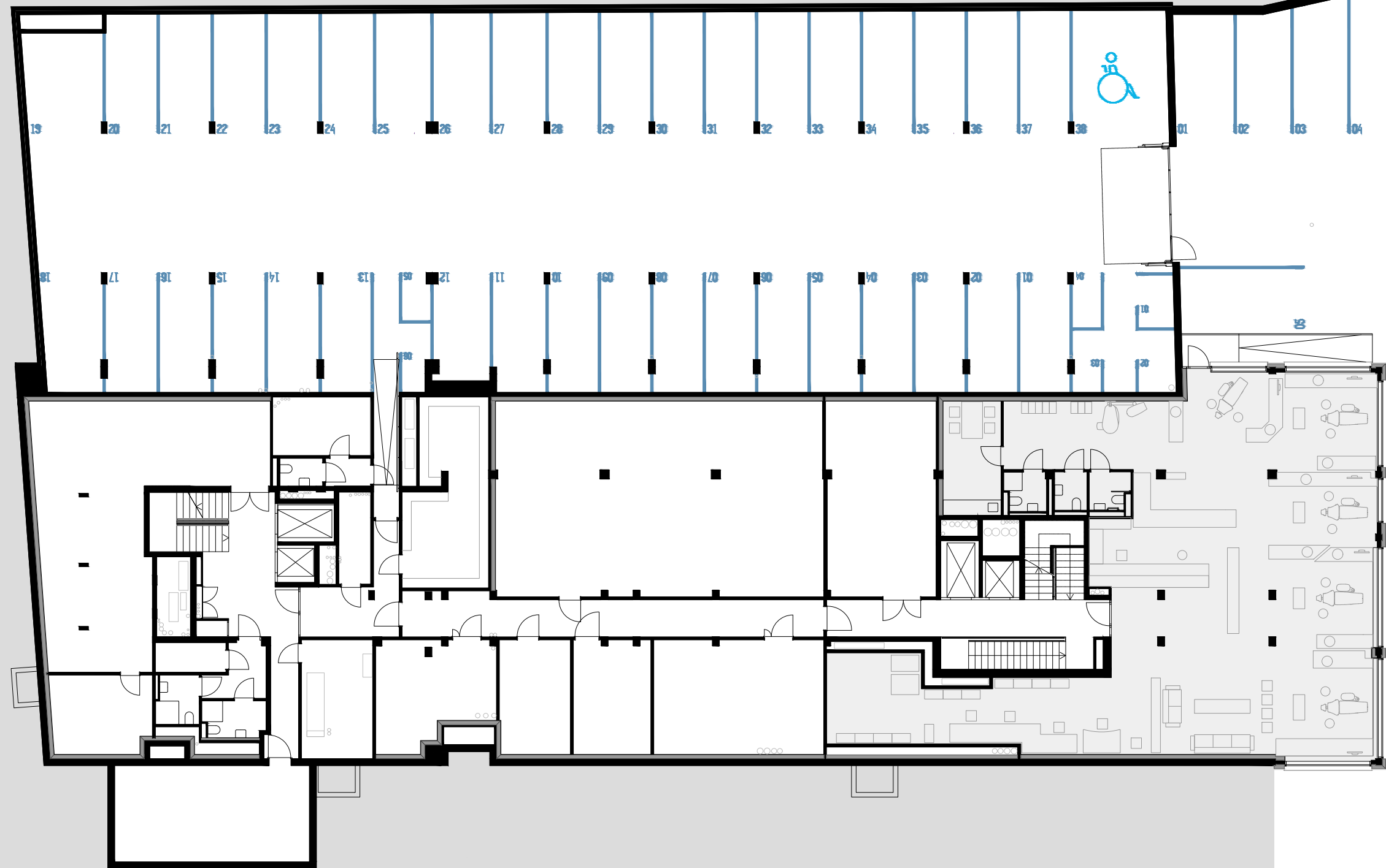
Plan du 1er sous-sol - entrée boulevard de Grancy
