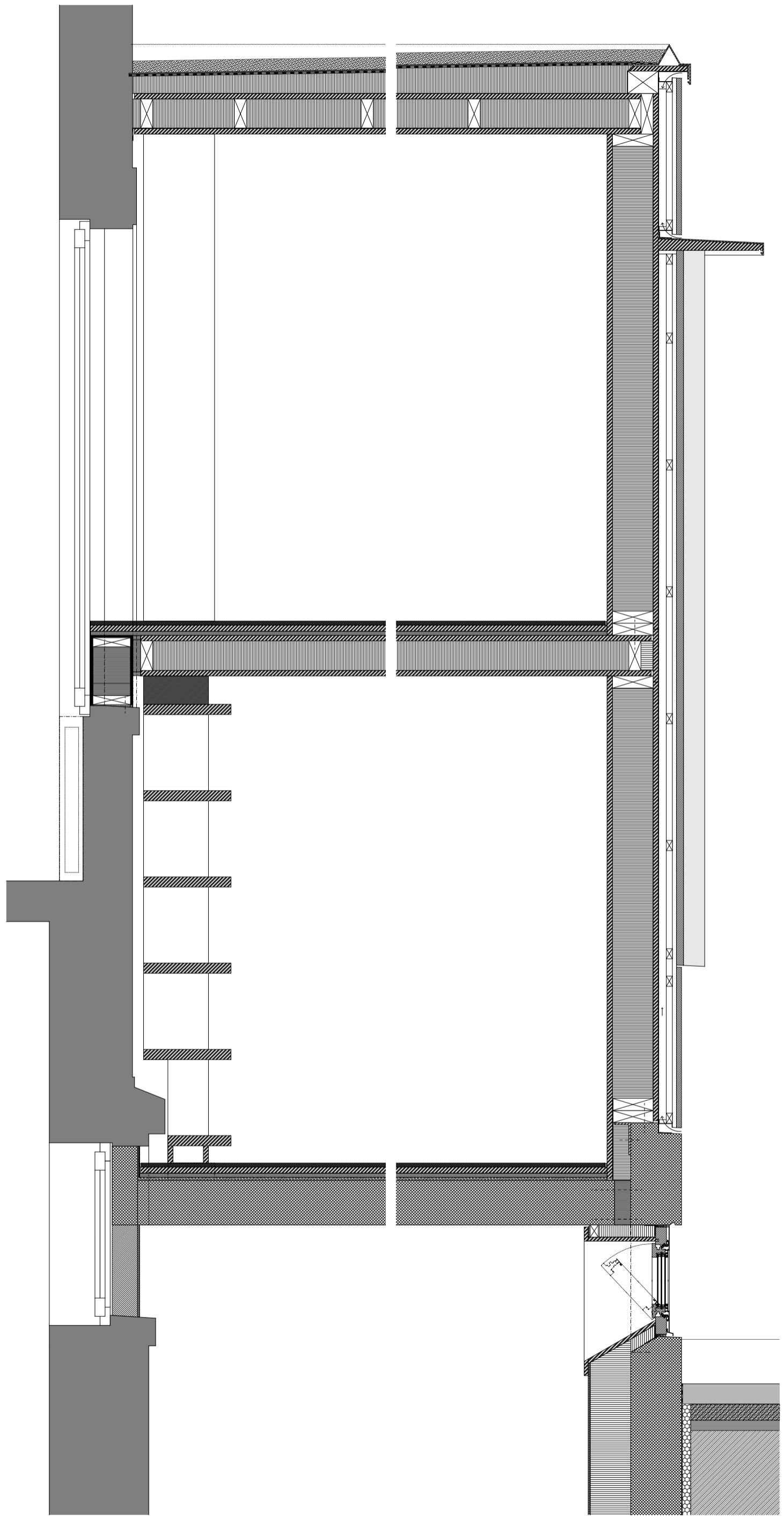
Fassadenschnitt 1:20
