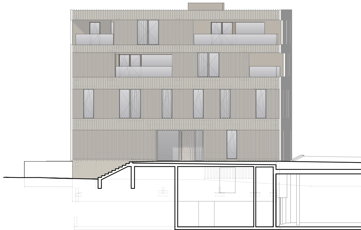
Fassade Süd-West 1:200
