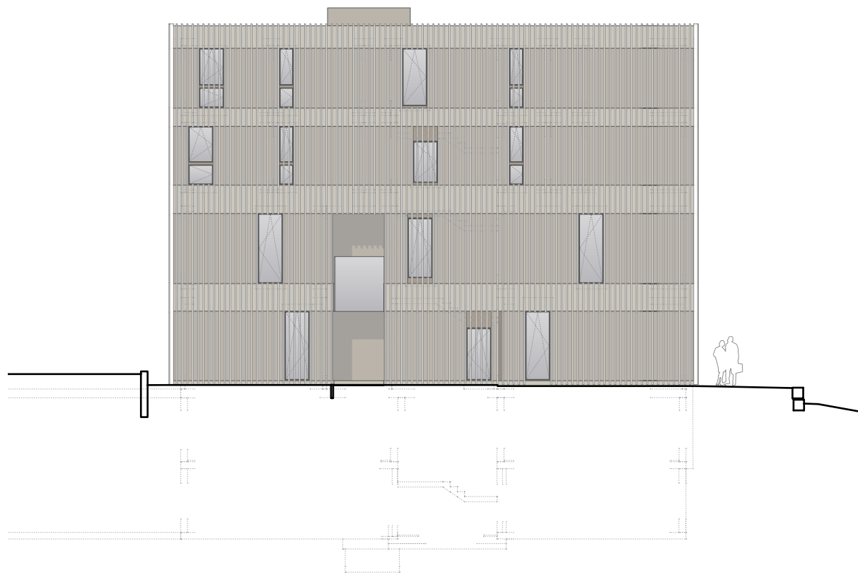
Fassade Nord-Ost 1:200
