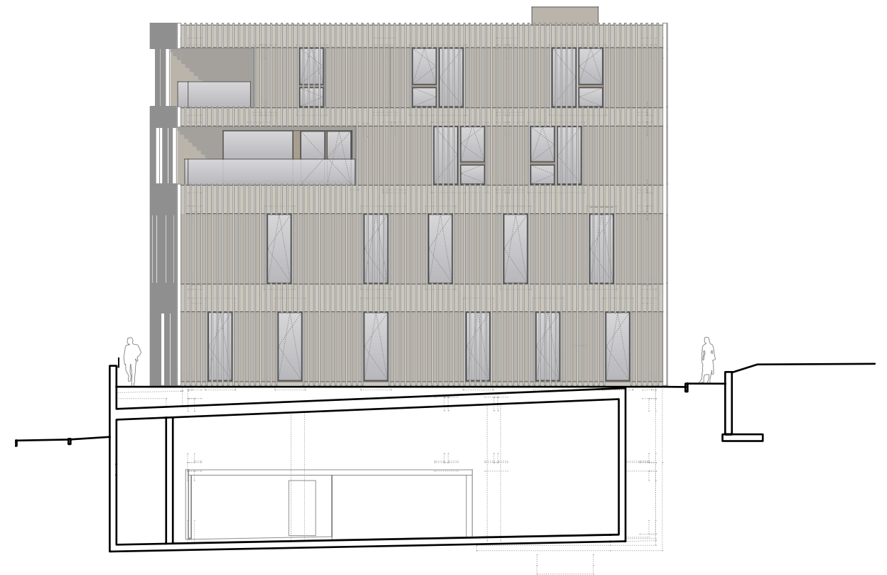
Fassade Süd-Ost 1:200
