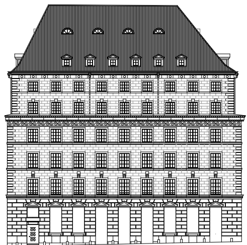
Ansicht Pelikanstrasse M1:500
