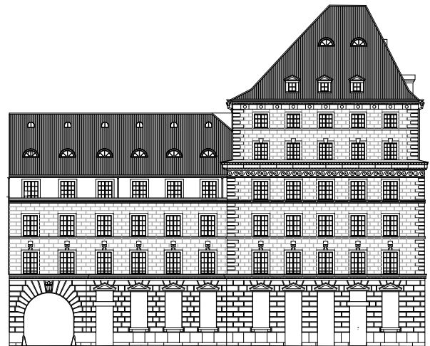
Ansicht St. Annagasse M1:500
