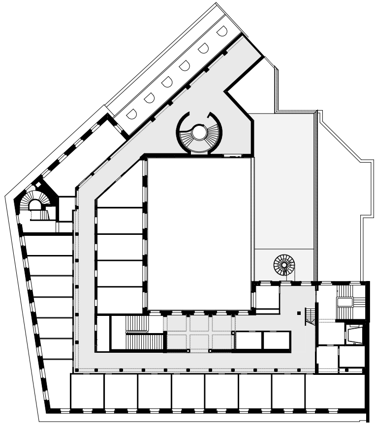
5. Obergeschoss M1:500
