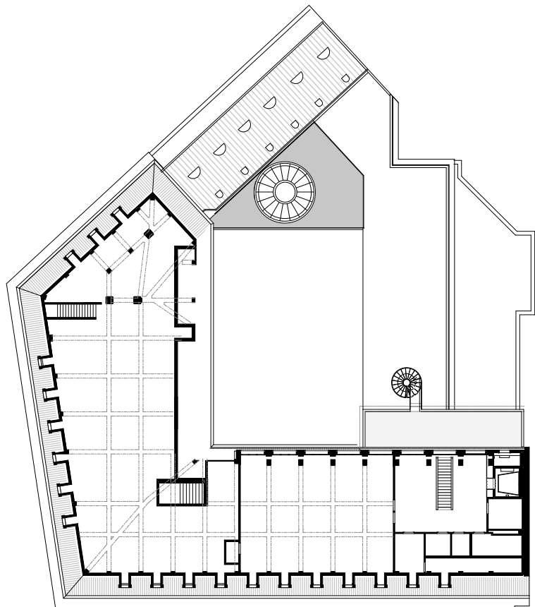
Dachgeschoss M1:500
