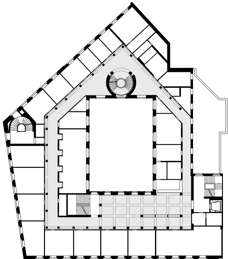
2. Obergeschoss M1:500
