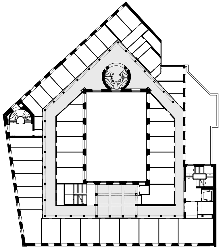
1. Obergeschoss M1:500
