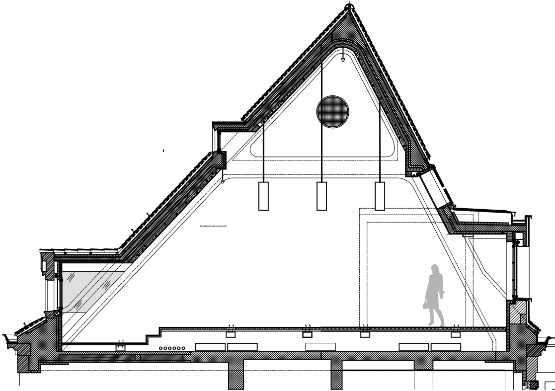
Detailschnitt Dach M1:100
