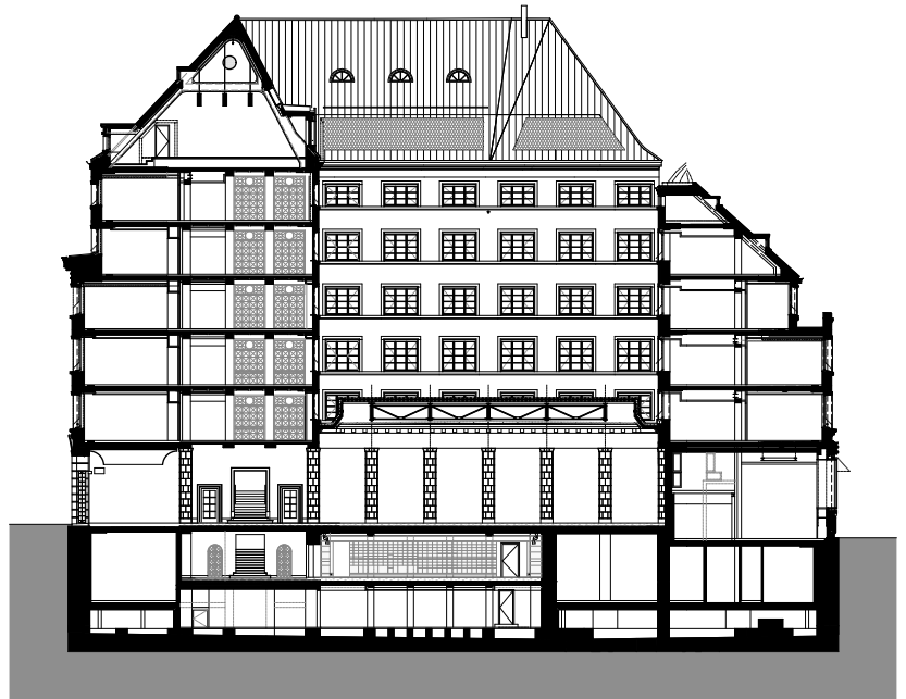
Schnitt A-A M1:500
