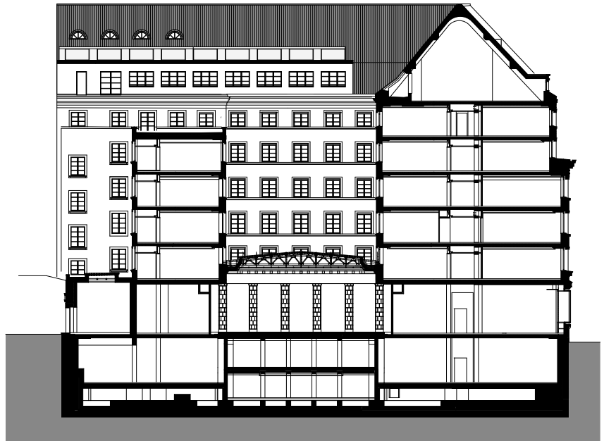
Schnitt B'-B' M1:500
