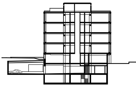
Querschnitt A, M 1:700
