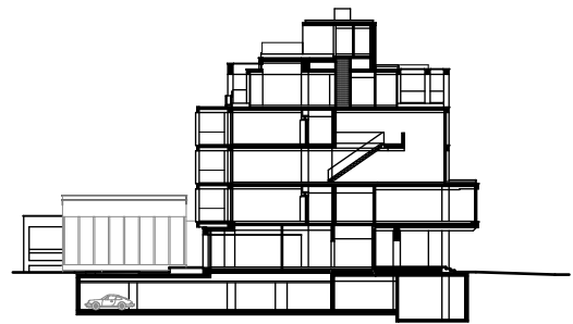
Querschnitt B, M 1:700
