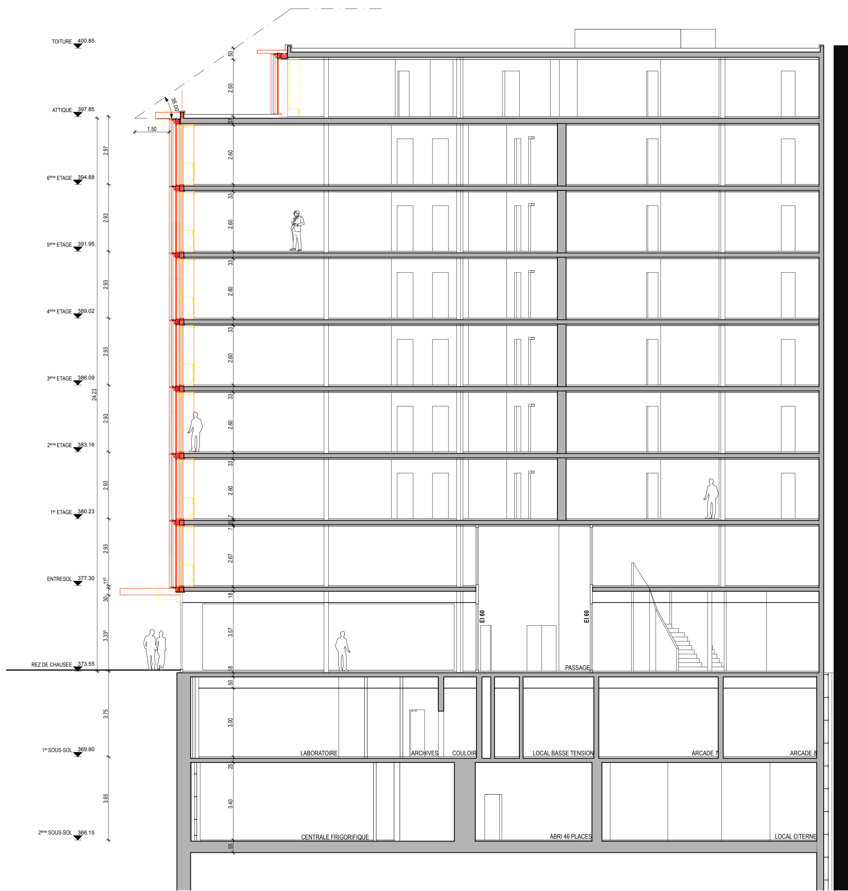
COUPE A
