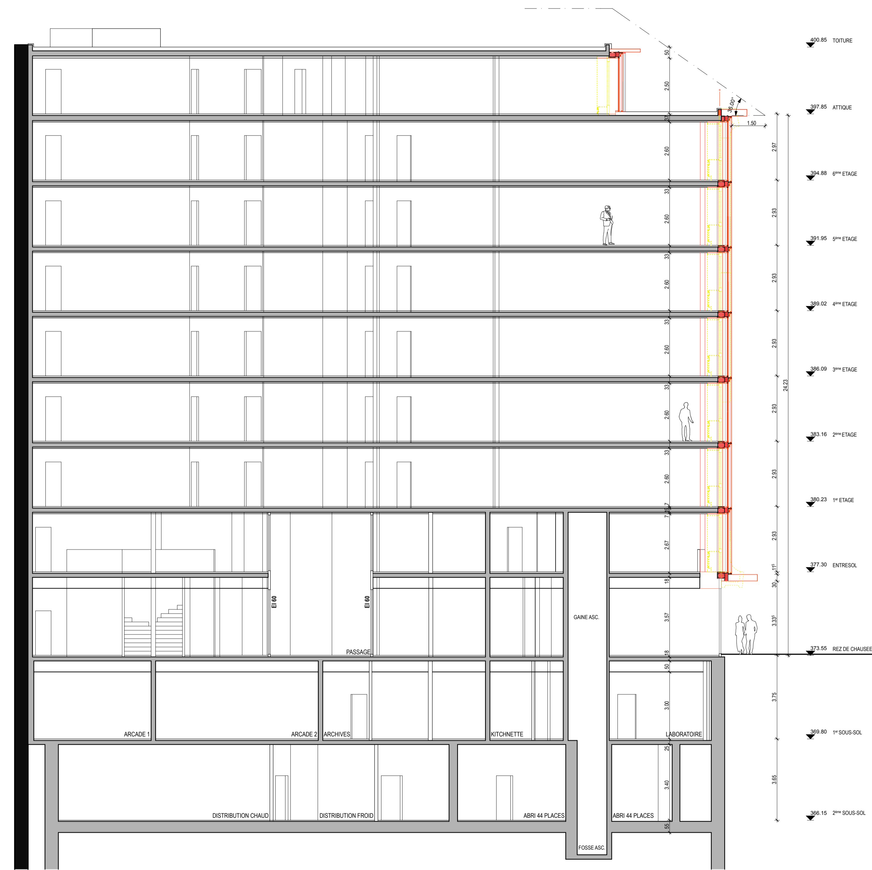
COUPE B
