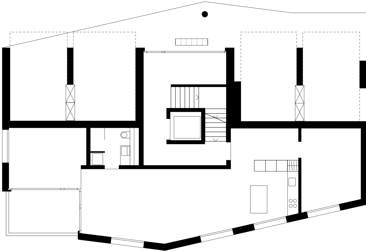
Grundriss EG 1:100
