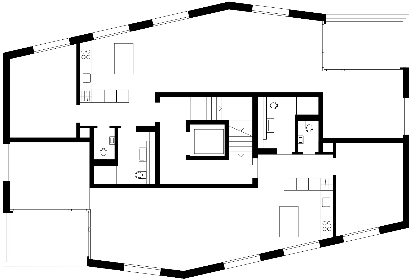
Grundriss OG 1:100
