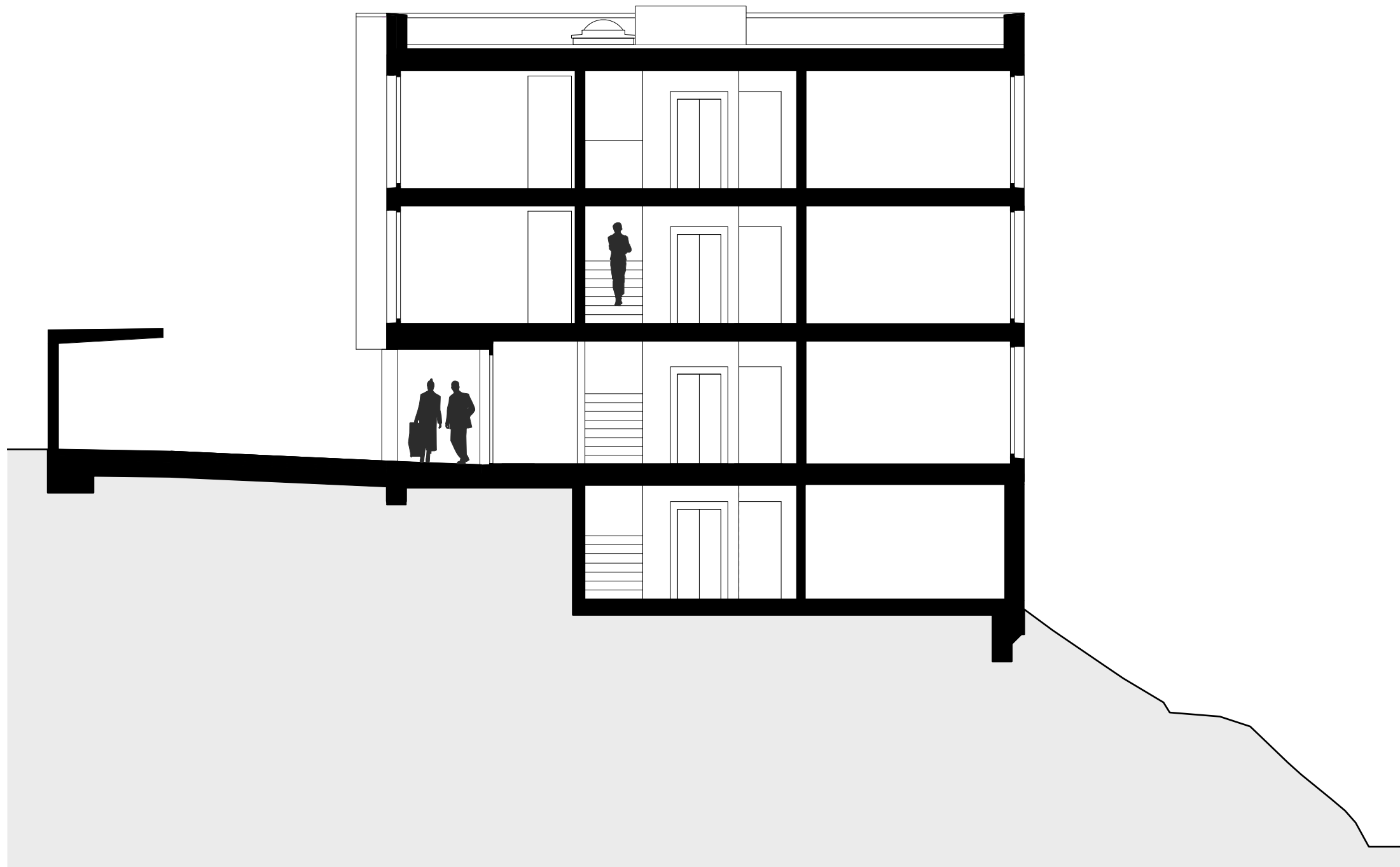
Querschnitt 1:100
