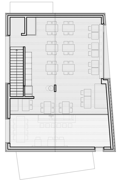
OBERGESCHOSS 1:200
