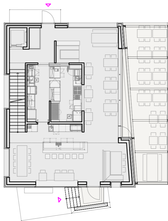
ERDGESCHOSS 1:200
