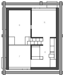
Obergeschoss 1:200
