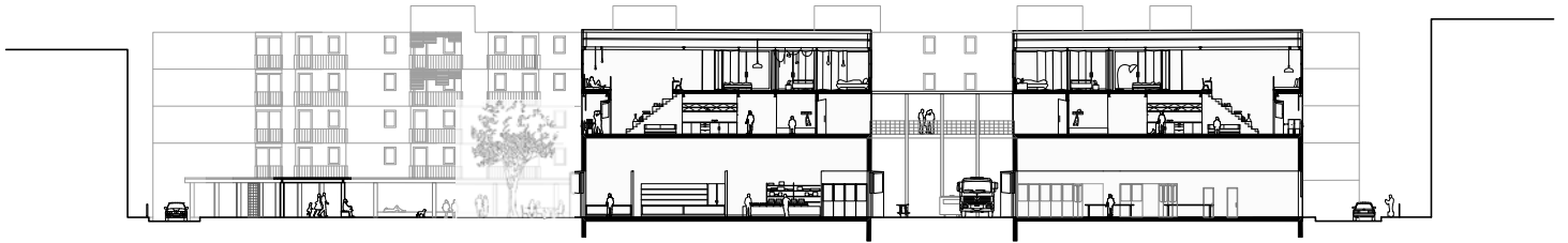
SCHNITT B 1/200
