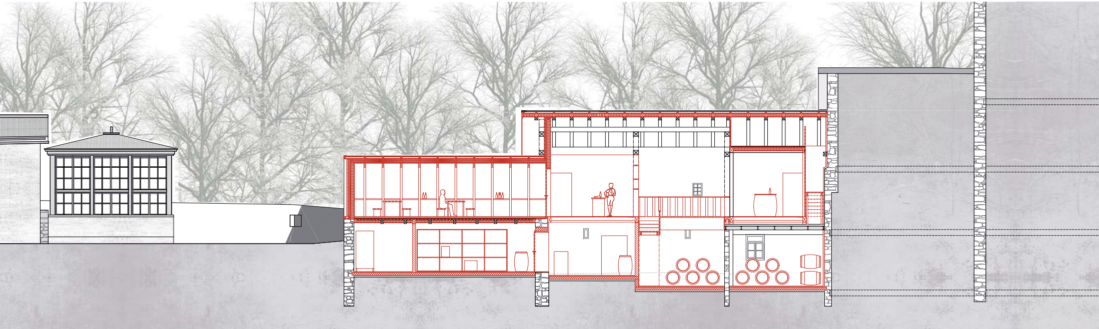
LÄNGSSCHNITT A, MST. 1:50
