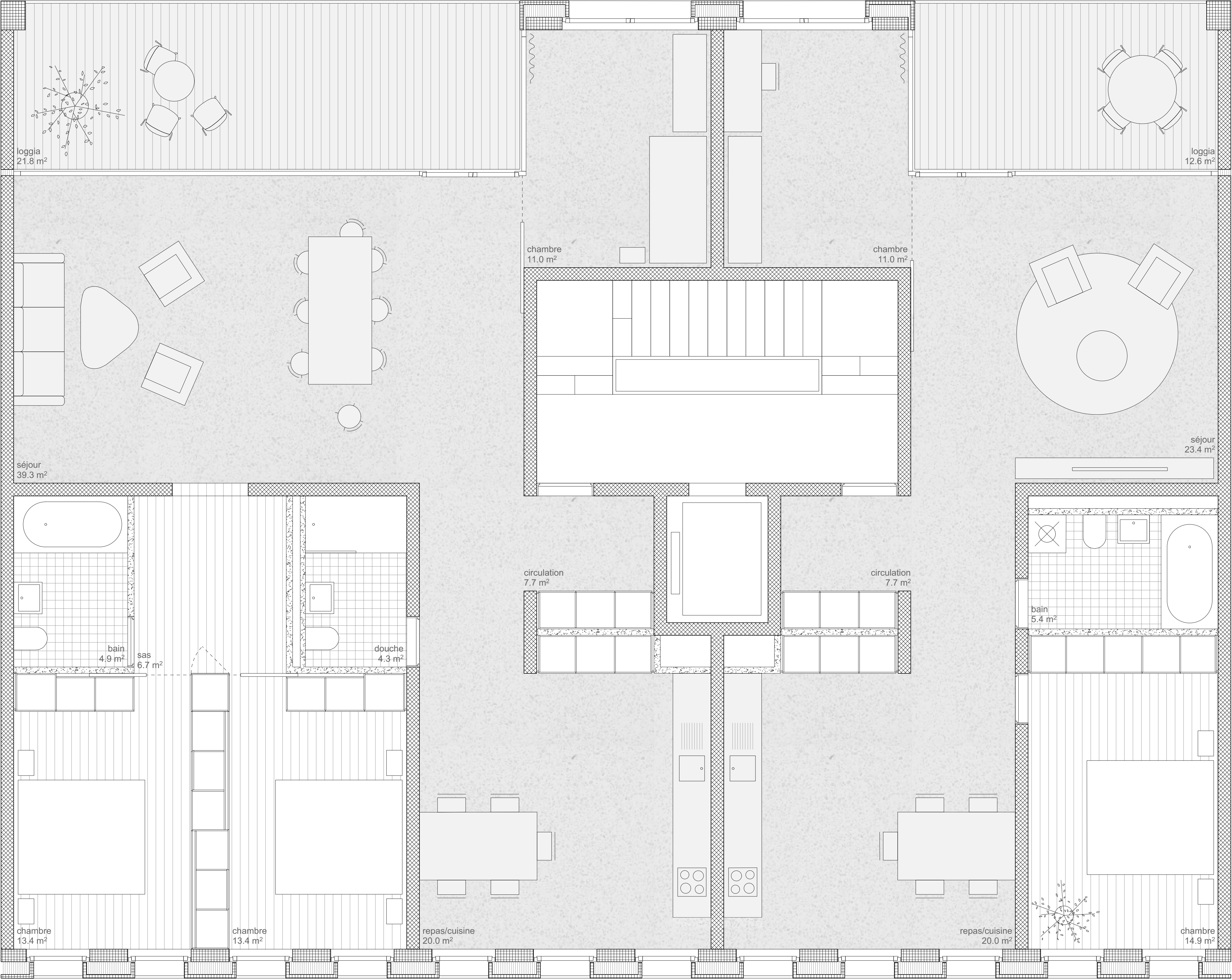
appartement type 1:33
