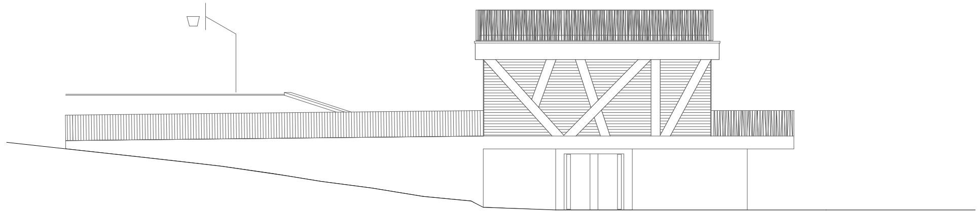
façade sud-est
