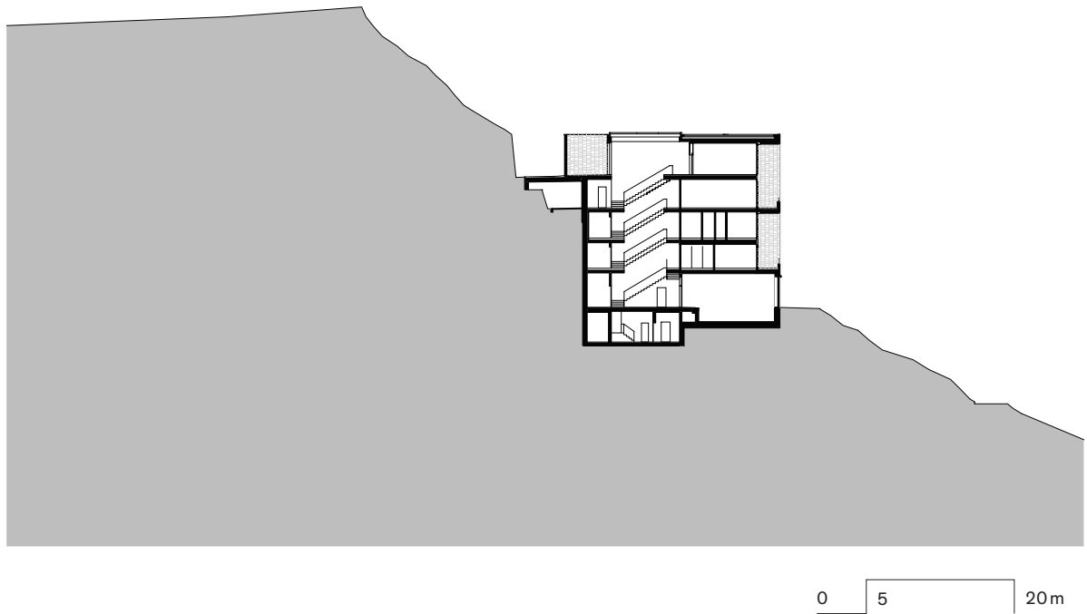
Situation und Querschnitt Rigi-Villa
